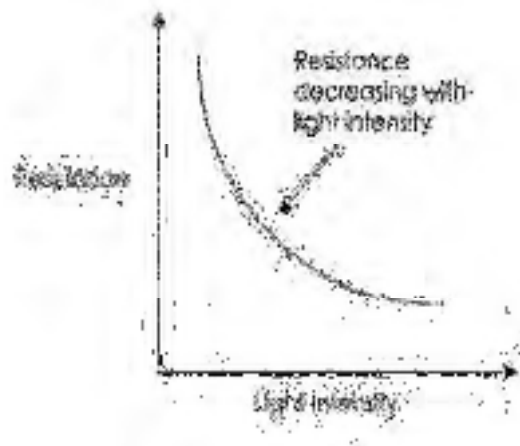
Gambar 2.15 Kurva pengaruh intensitas cahaya terhadap LDR.
