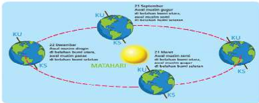
Gambar 2.5: Rotasi Bumi terhadap Matahari
