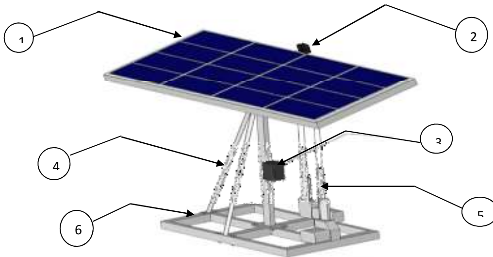
Gambar 3.1 : Double axis
