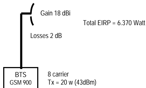
Gambar 6. EIRP yang dipancarkan oleh antenna BTS
